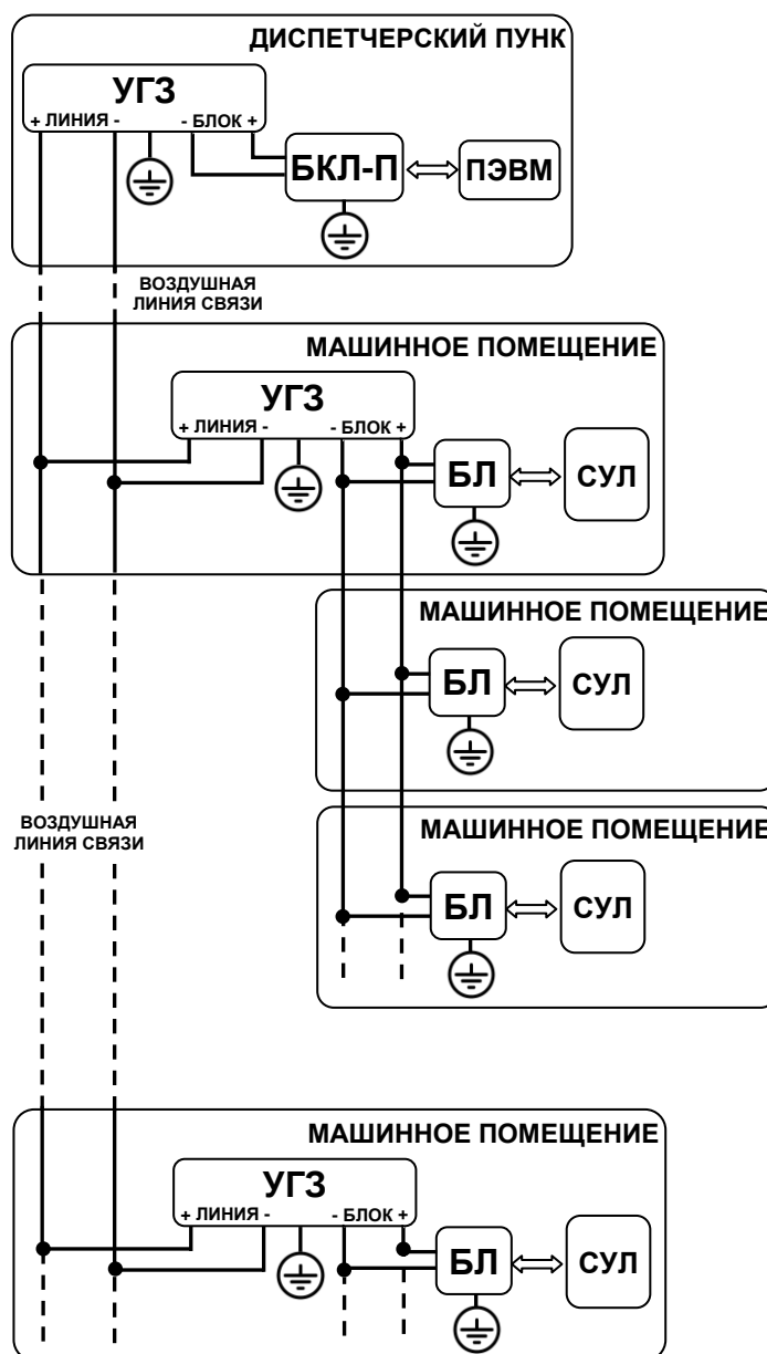
Рис.2 Схема подключения Устройство грозозащиты УГЗ-60В-0,25А НШЕК.468243.006
