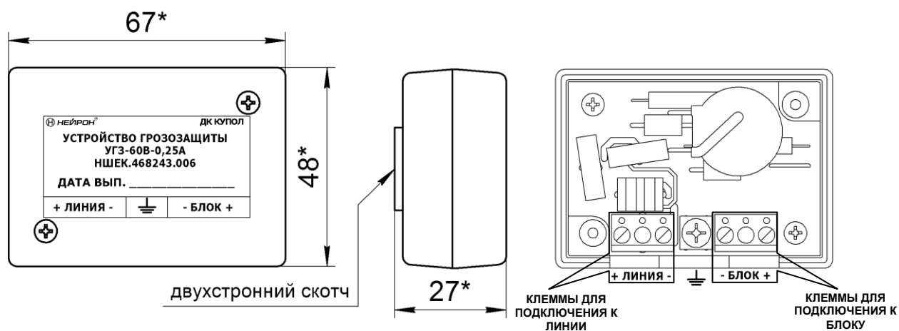
Рис.1 Внешний вид Устройство грозозащиты УГЗ-60В-0,25А НШЕК.468243.006
